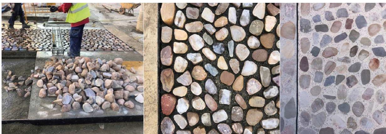
Imágenes del proceso de ejecución del empedrado tradicional recuperado
